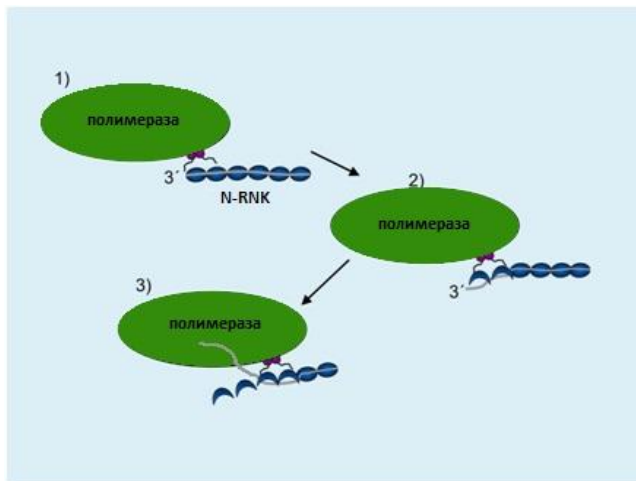
Слика 1.3. Претпостављени модел активности ензима полимеразе
