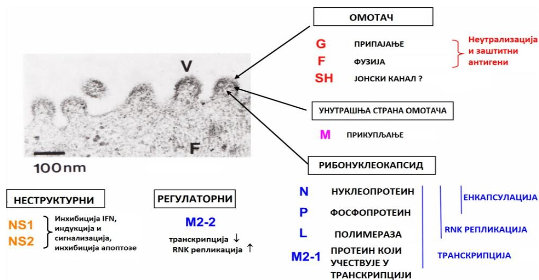
Слика 1.1. Грађа RSV вируса (према референци Collins and Melero, 2011)
