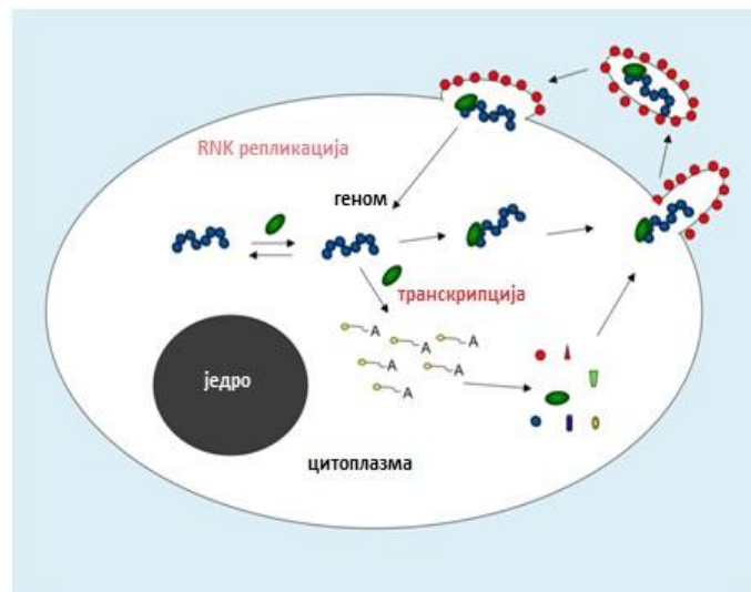
Слика 1.2. Циклус RSV репликације
